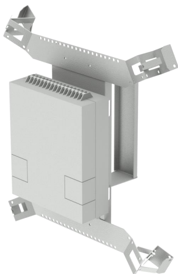
wizualizacja stelaża zapasu kabla SZK-K z akcesoriami
