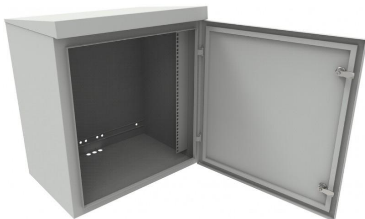
wizualizacja otwartej szafy masztowej rack 19" hermetycznej serii SZMH
